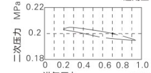
适用型号: GR600
