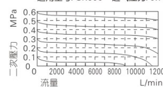
适用型号: GR600 进气压力: 0.7MPa
