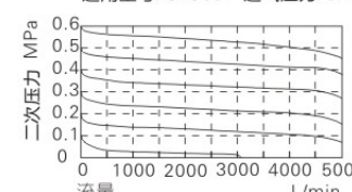
适用型号: GR300 进气压力: 0.7MPa
