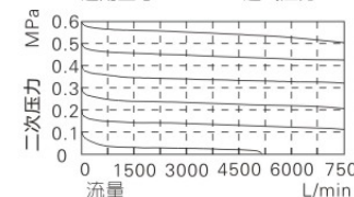
适用型号: GR400 进气压力: 0.7MPa
