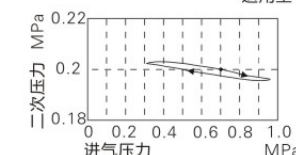
适用型号: GR600
