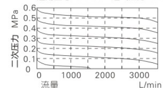
适用型号: GR200 进气压力: 0.7MPa
