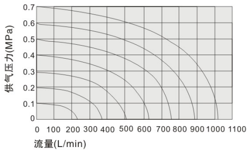
4YV110-06流量图
