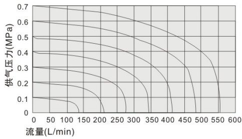
4YV110-M5流量图
