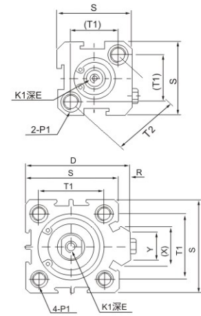
外牙尺寸
