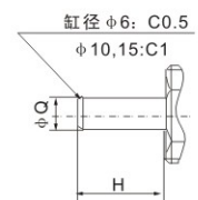
杆端无螺纹情况
